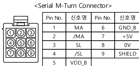
Plug : 172169-1(AMP)
