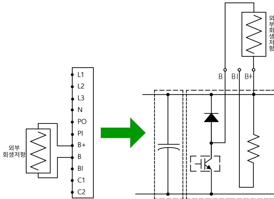
외부 회생 저항 사용 시 배선 방법
