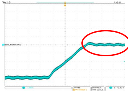
출력 오프셋: 1000 rpm 출력 스케일: 500rpm/V
