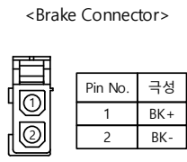
Plug : 172165-1(AMP)
