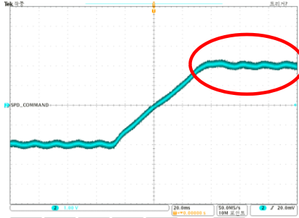
출력 오프셋: 0 rpm 출력 스케일: 500rpm/V
