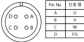
Plug : MS3102A22-22P
