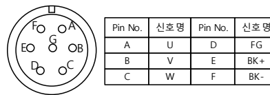
Plug : MS3102A20-15P
