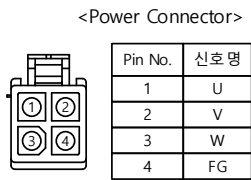
Plug : 172167-1(AMP)
