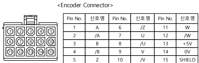
Plug : 172171-1(AMP)
