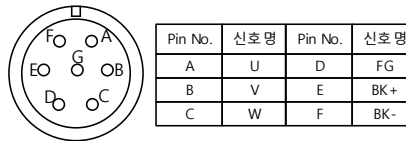
Plug : MS3102A24-10P
