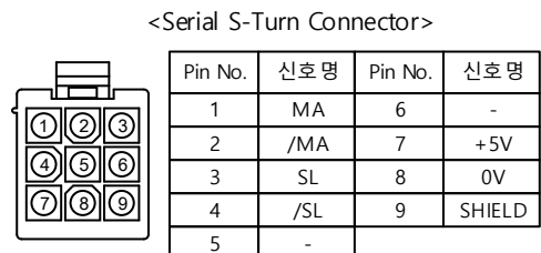
Plug : 172169-1(AMP)
