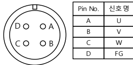
Plug : MS3102A20-4P
