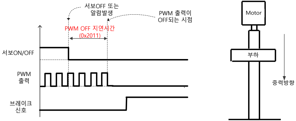
(2) PWM 출력이 먼저 OFF 되고 브레이크 신호가 출력되는 경우
