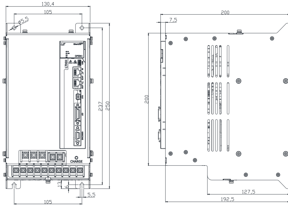
*중량 : 5.5[kg] (냉각팬 포함)
