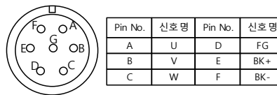
Plug : MS3102A20-15P
