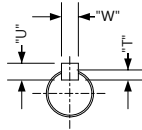
(축단 치수 상세도)
