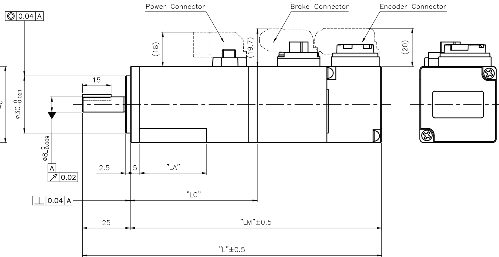
<외형 치수>
